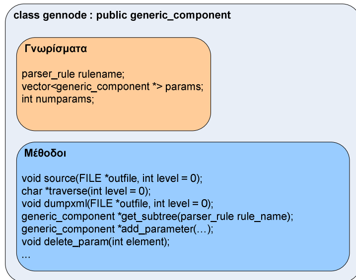
Σχήμα 4.8 Η κλάση gennode
