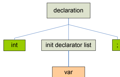
Σχήμα 4.13 Υπόδεντρο δήλωσης μεταβλητής
