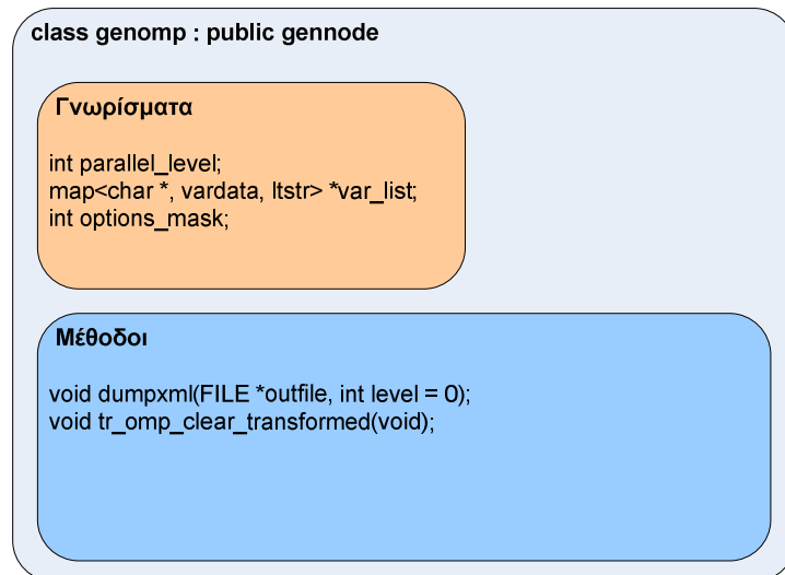
Σχήμα 4.14 Η κλάση genomp
