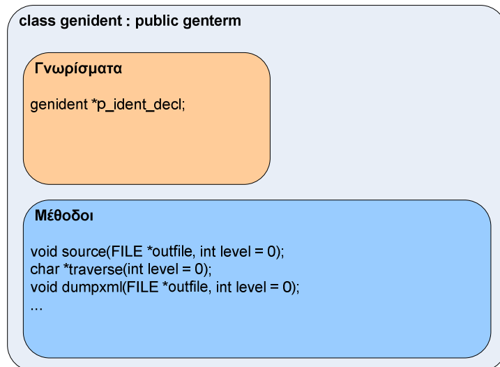
Σχήμα 4.7 Η κλάση genident
