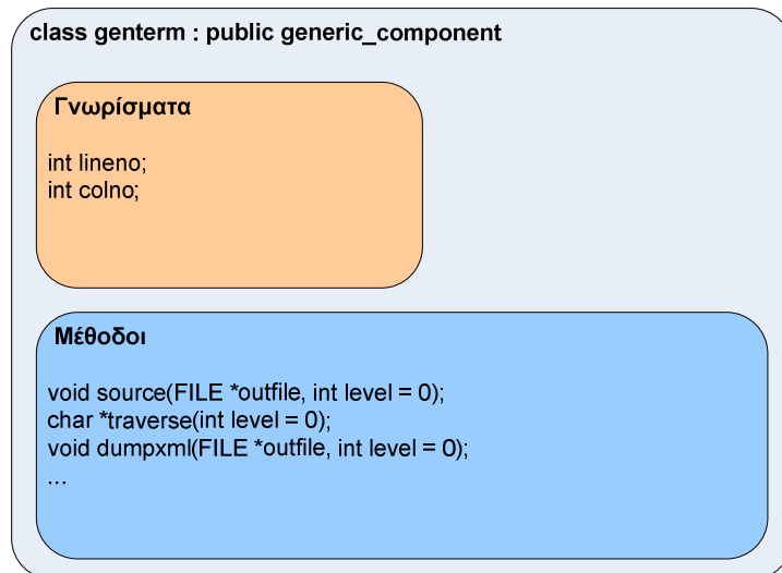
Σχήμα 4.6 Η κλάση genterm
