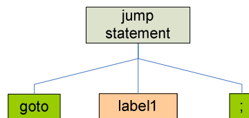
Σχήμα 3.1 Παράδειγμα κατασκευής υποδέντρου
