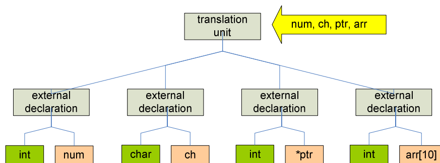
Σχήμα 3.2 Απλοποιημένο παράδειγμα χάρτη μεταβλητών
