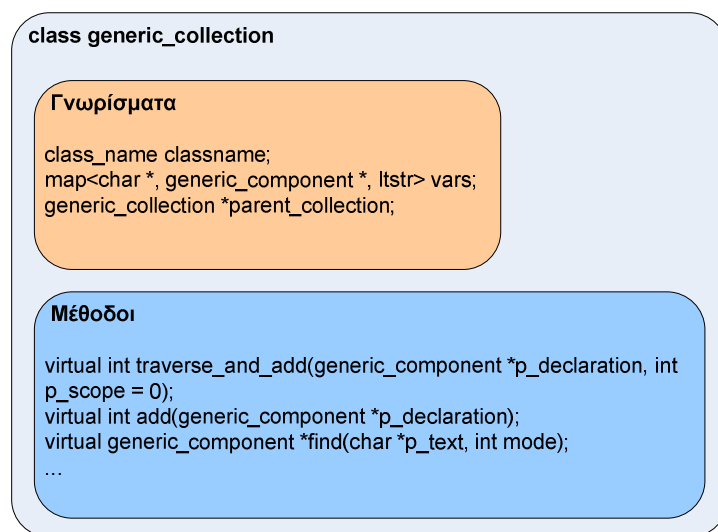
Σχήμα 4.15 Η κλάση generic_collection
