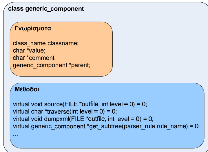
Σχήμα 4.5 Η κλάση generic_component
