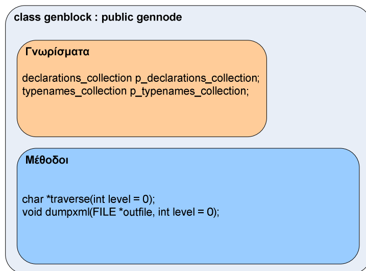
Σχήμα 4.10 Η κλάση genblock
