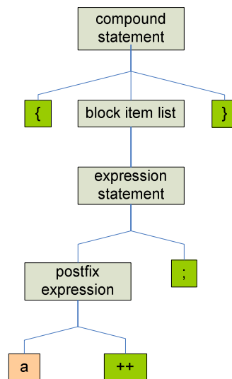
Σχήμα 4.11 Απόσπασμα του ΣΣΔ
